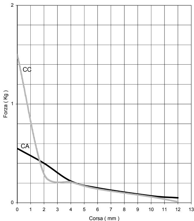
PRESTAZIONE ELETTROMAGNETE
