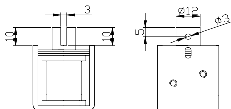
VERSIONE A TRAZIONE
