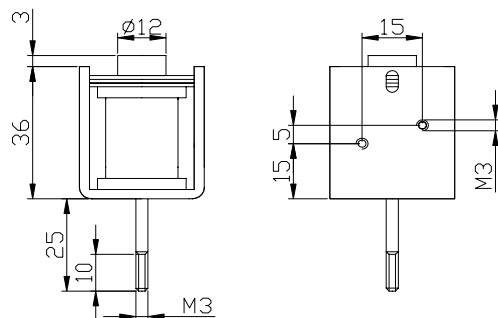
VERSIONE A TRAZIONE
